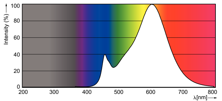
2700 K, 470 lm
