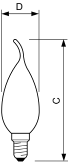
filament 2.5W-25W 250lm NAD 2700K E14ND
